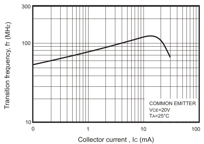
Fig.6- f_T - I_c
