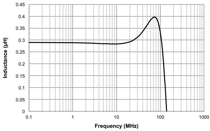
MPI4012V2-R33-R
