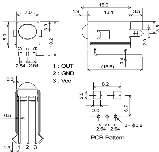
NJL74H000A UNIT:mm
