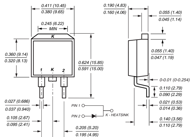
TO-263AB (NSBxT)
