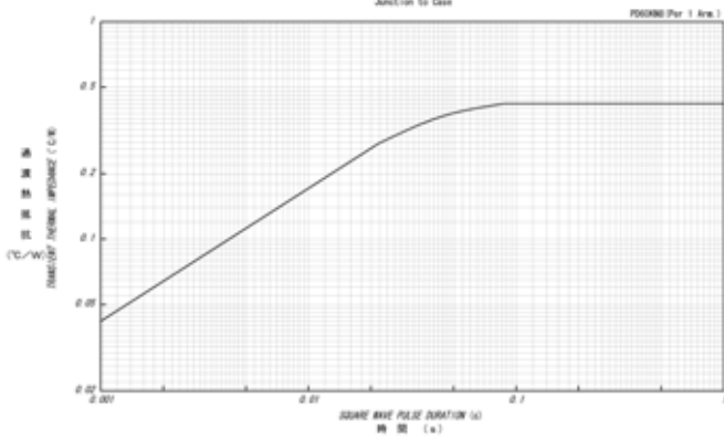
過渡熱抵抗特性 RULDER TRANSIENT THERMAL IMPEDANCE
