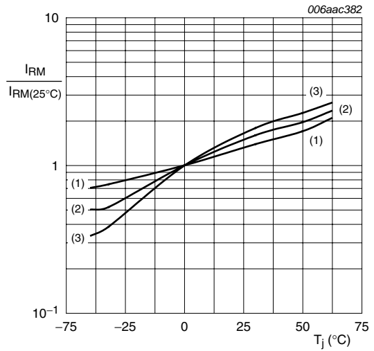
(1) PESD3V3V4UK (2) PESD5V0V4UK (3) PESD9V0V4UK
