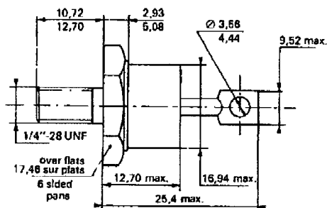
DO-5 (CB-34)
