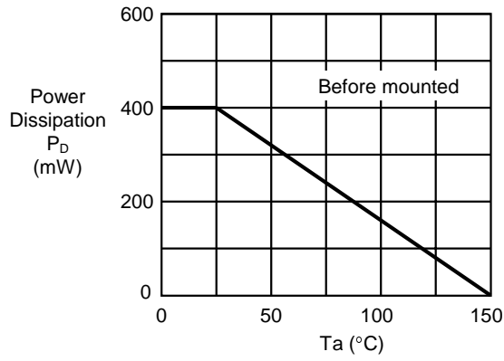
(1) TO-92
