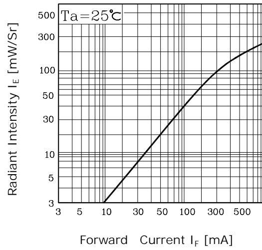
Fig. 2 I_E - I_F
