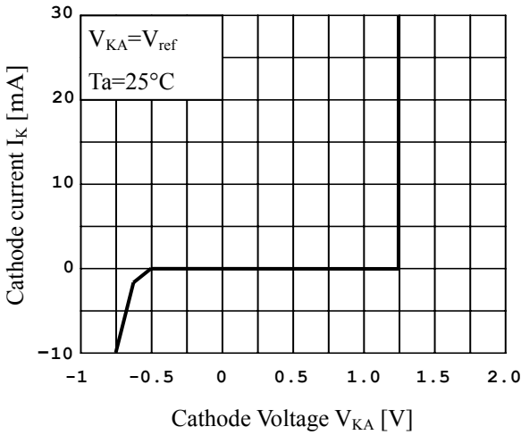
Fig.4 I_K vs V_{KA} (1)
