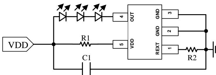
图 2. SM1501 典型应用电路
