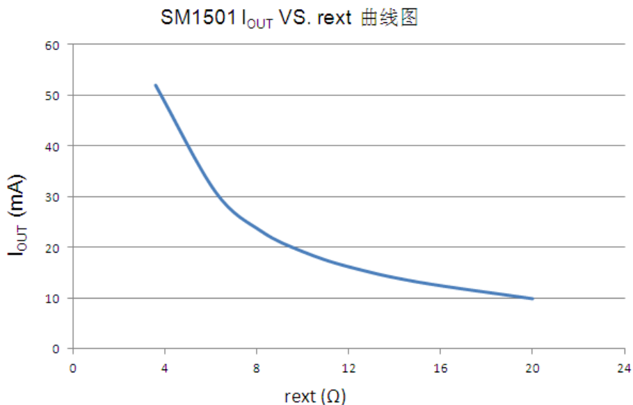
图 3. SM1501 输出电流与 REXT 电阻关系曲线
