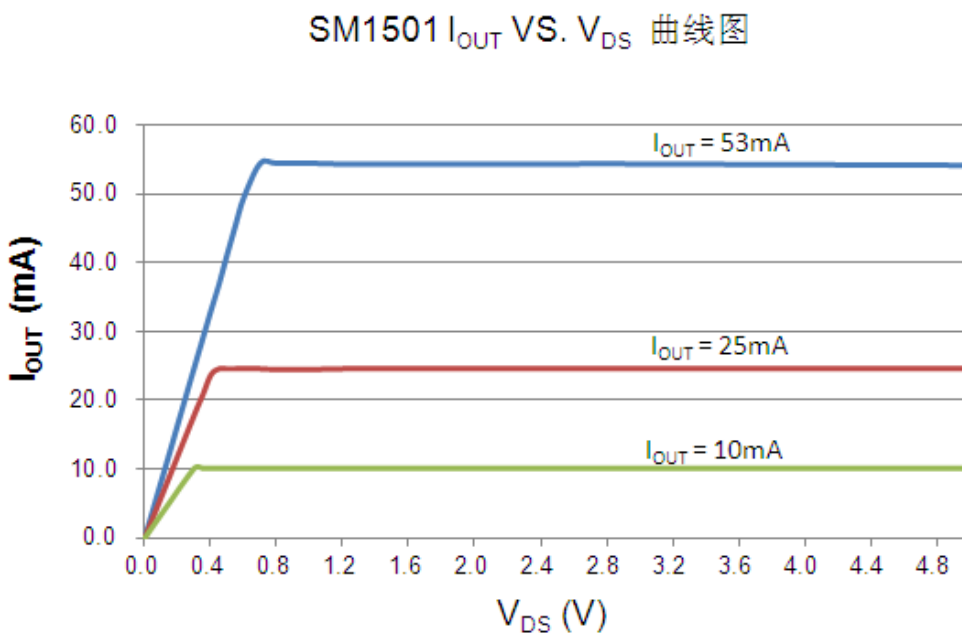
图 4. SM1501 输出电流与 OUT 端口电压 V DS 关系曲线 测试条件：VDD = 5.0V
