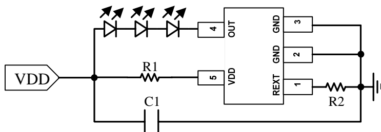
图 7. SM1501 典型应用电路
