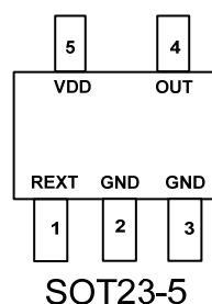
图 1. SM1501 各封装脚位图
