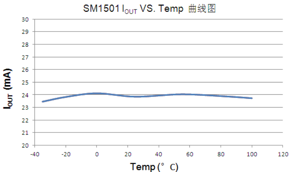
图 5. SM1501 恒流电流对温度变化曲线图
