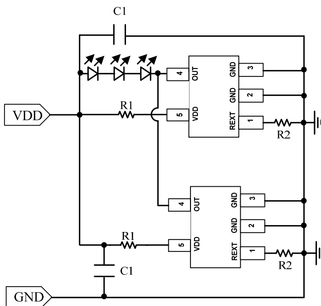
图 8. SM1501 并联应用电路原理图
