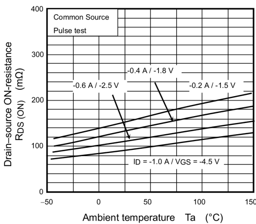
Fig. 7.1.5 R_{DS(ON)} - T_a
