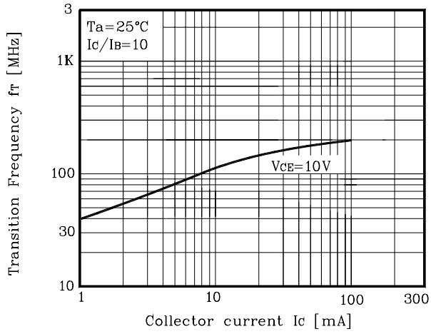
Fig. 7 f_T - I_C
