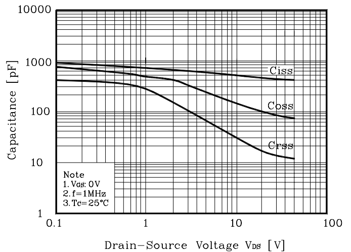
Fig. 6 Capacitance - V_{DS}
