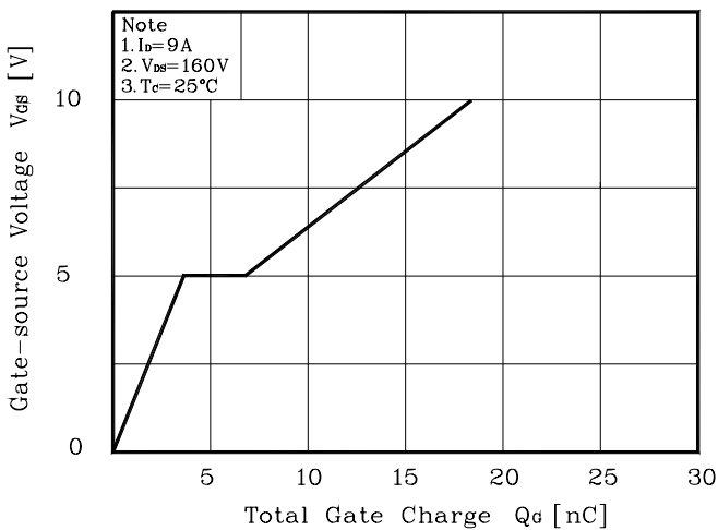
Fig. 5 V_{GS} - Q_G
