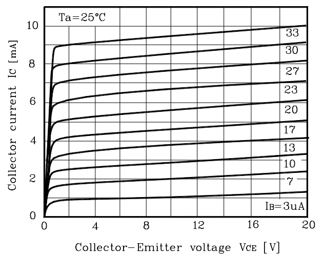
Fig. 2 I_C - V_{CE}
