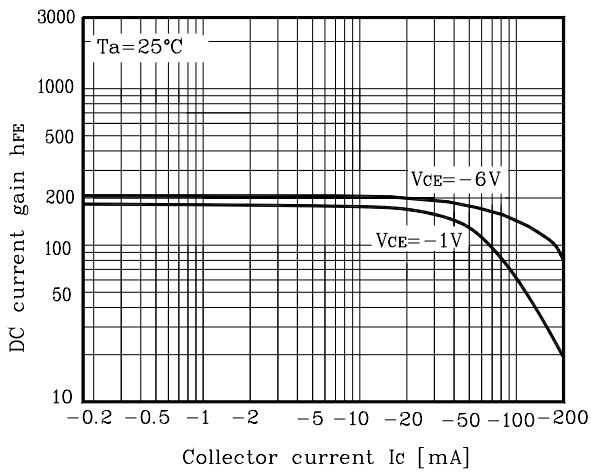
Fig. 3 h_{FE}-I_C
